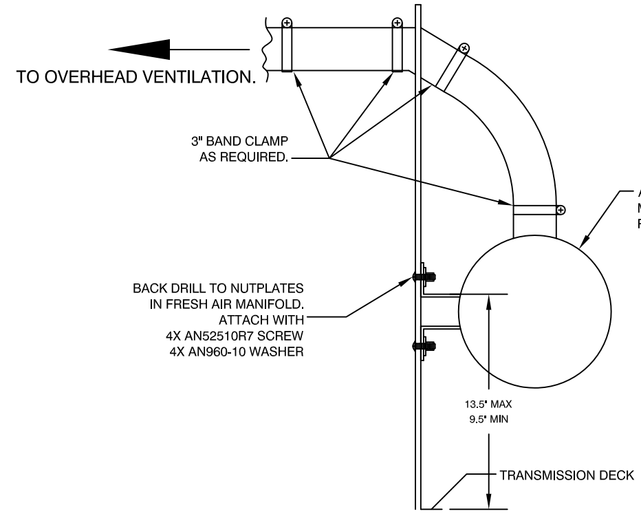
VIEW A-A
